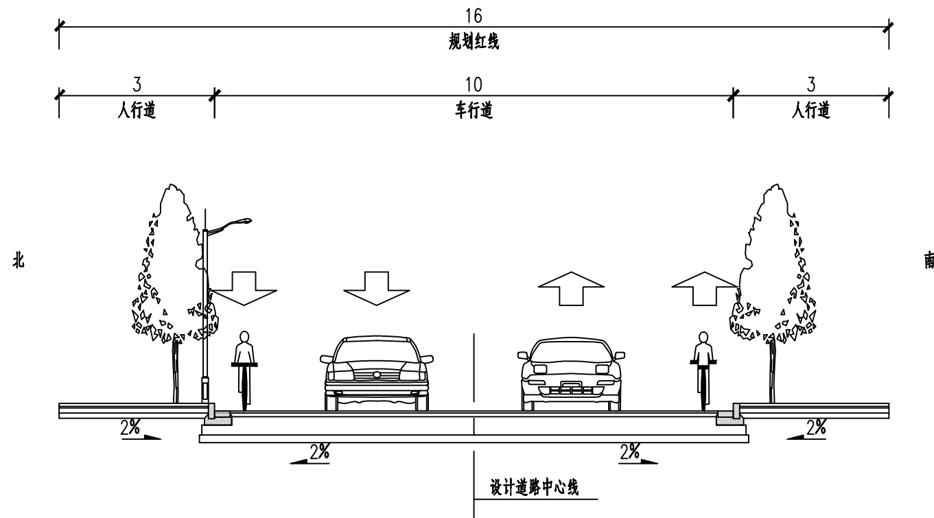
李塔东街(酬勤南路-辰塔路)标准横断面设计图
